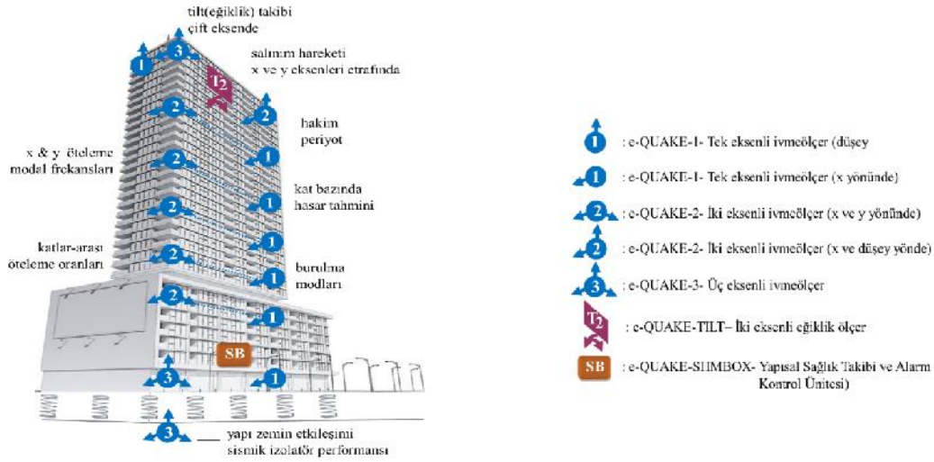
ekil 4. Binalarda Yapısal Sağlık Takibi - Parametreler ve enstrüman yerleşim özeti
