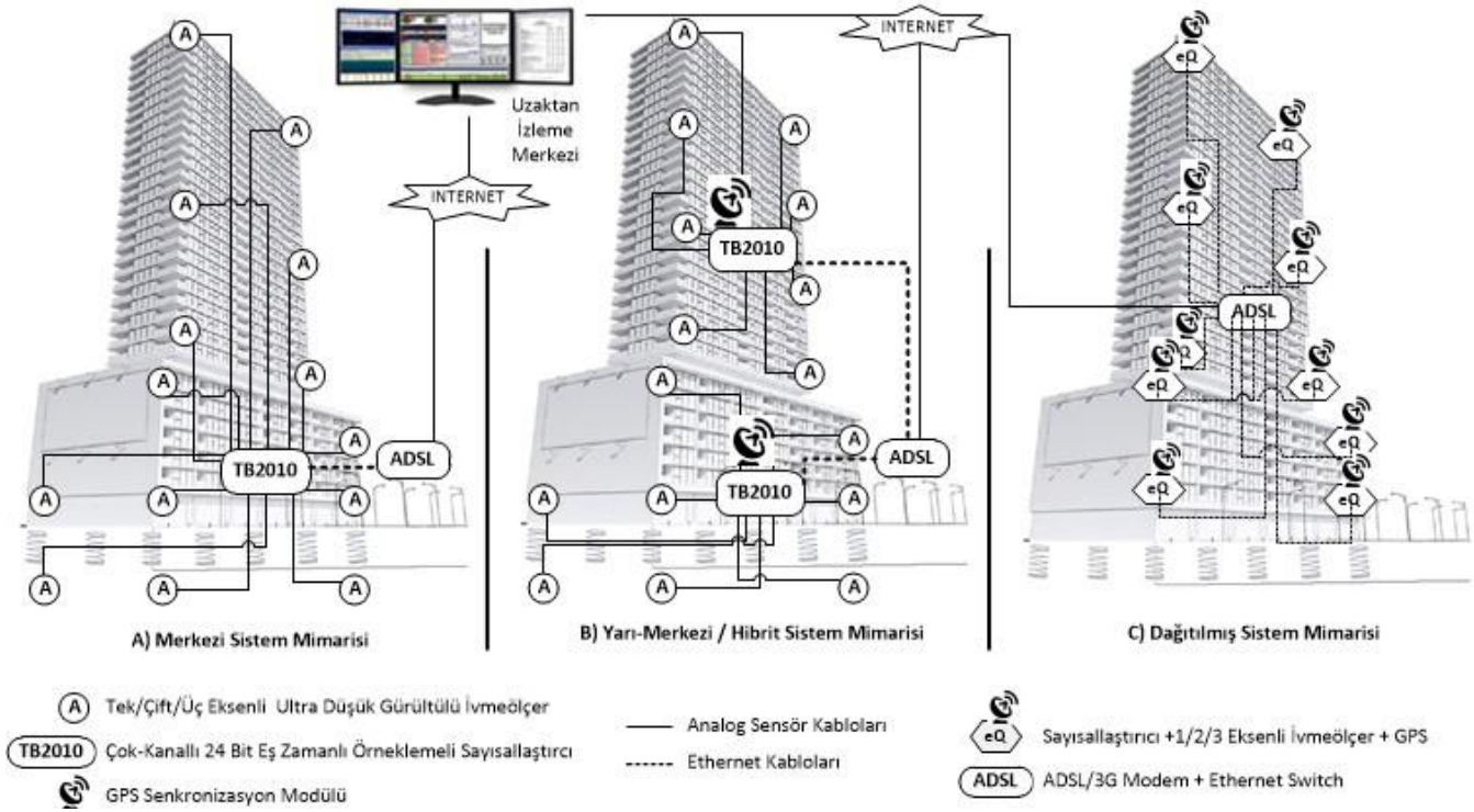
ekil 8. Yapısal Sağlık Takibi Farklı Yerleşim Mimarileri
