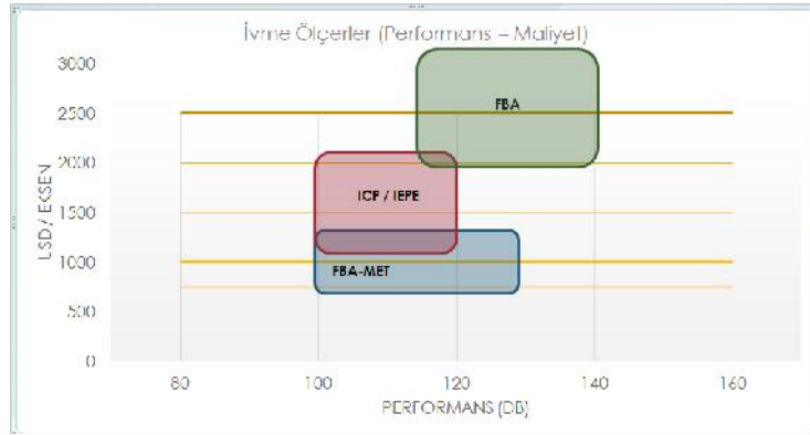
ekil 5. vmeölçer tiplerine göre performans/maliyet karşılaştırması
