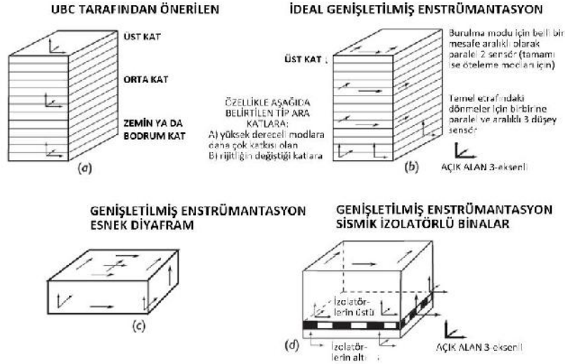
ekil 3. Binalarda ivmeölçer yerleşimi. Çelebi(2002)'nin, USGS(Birleşik Amerika Jeolojik Araştırmalar Kurumu) için hazırladığı rapordan Türkçeleştirilerek alıntılanmıştır.
